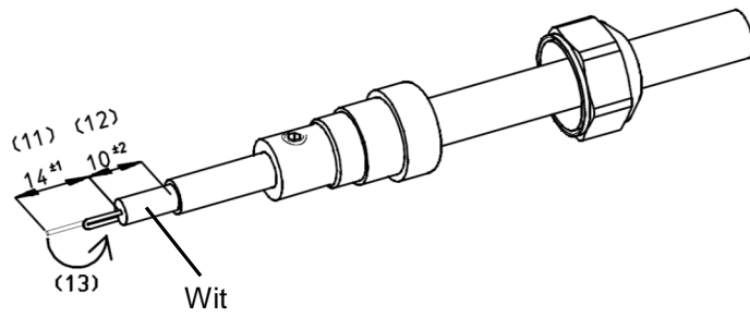
Afbeelding 3: afwerking coaxkabel
