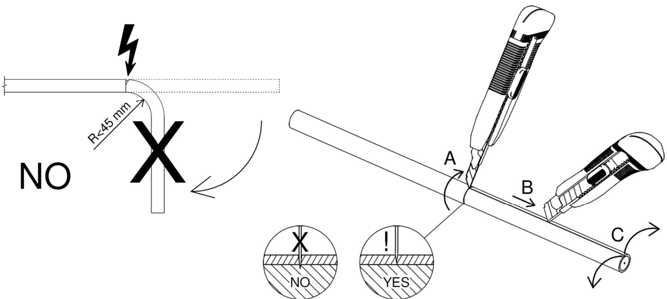
Afbeelding 2: kabelmantel strippen
