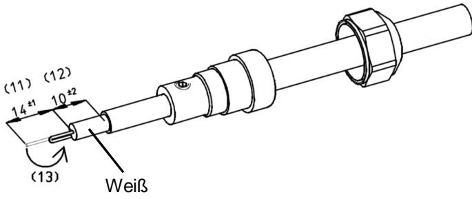
Abbildung 3: Abisolieren des Koaxialkabels
